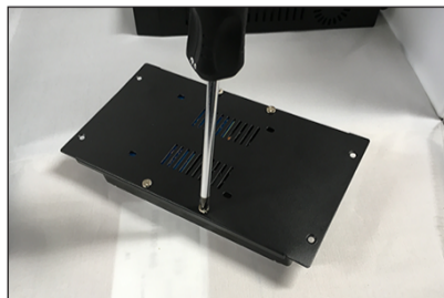
取り外した蓋にハードディスクをねじで取り付けます。
